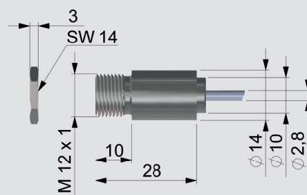
Dimensions optris CSmicro 2W
